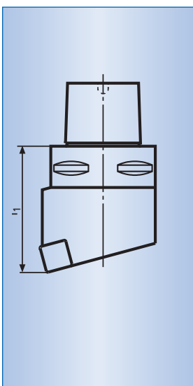
Werkzeuglänge Tool length Longueur d'outil
